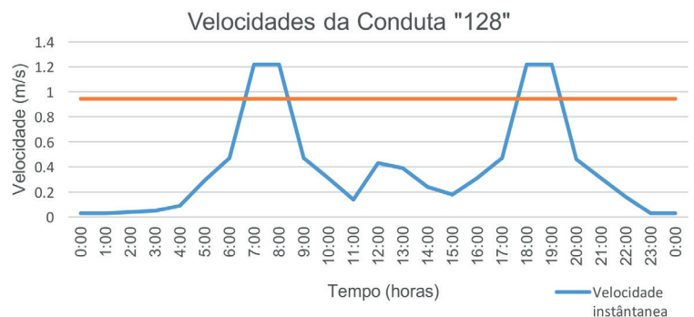
Figura 8. Excedências horárias à velocidade instantânea máxima da Conduta "128"
