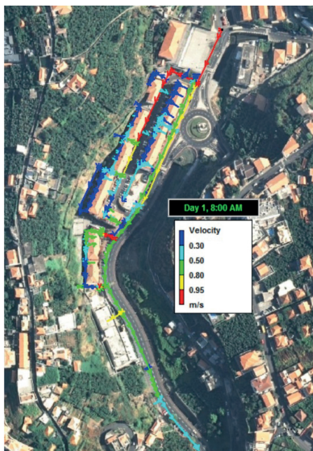
Figura 7. Distribuição espacial das velocidades à hora de maior consumo (08:00) no modelo alterado
