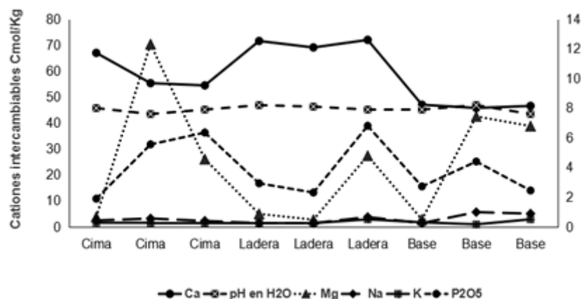
Fig. 2 - Contenido de macronutrientes en las muestras de suelo.
