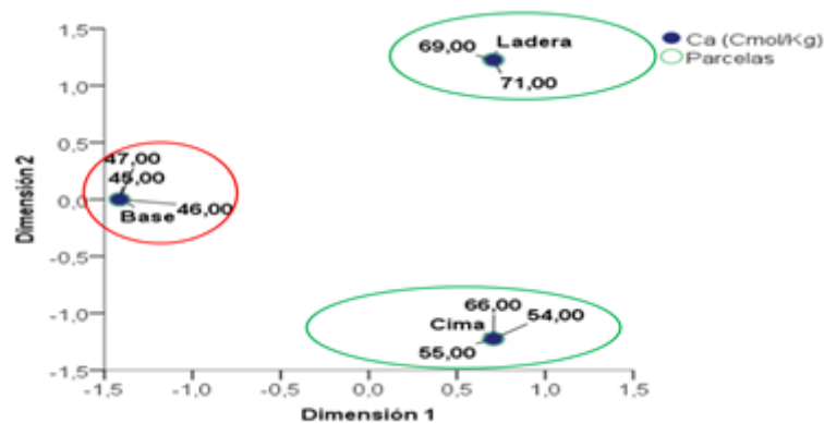
Fig. 3 - Representación de la relación entre concentraciones de Ca y los niveles topográficos.
