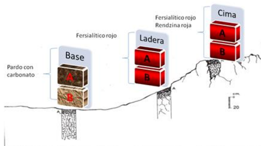
Fig. 4 - Tipos de suelo presentes en la superficie estudiada.
