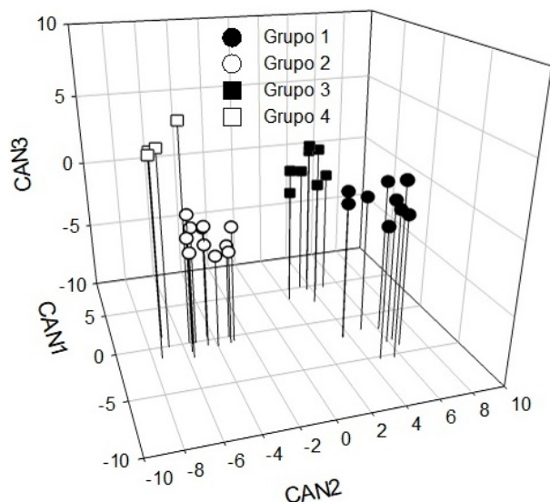
Figura 2. Representación tridimensional en las dos tres raíces canónicas de 32 genotipos de ciruela mexicana.
