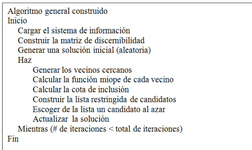
Figura 1: Procedimiento de búsqueda miope aleatorizado y adaptativo.
