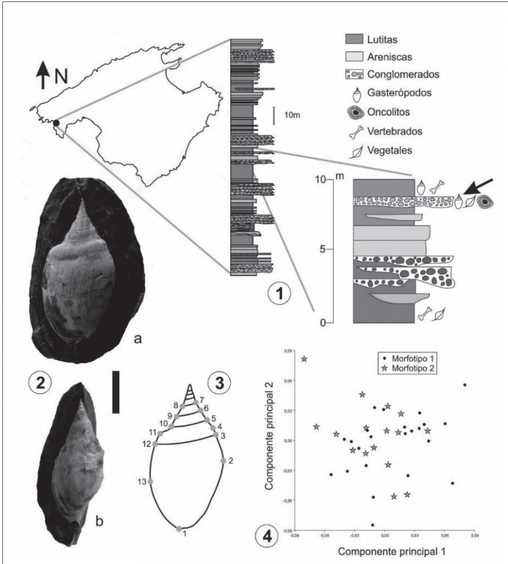
Figura 1. 1. Situación geográfica de la serie oligocena de la Serra des Gats y su contexto estratigráfico (adaptado de Ramos-Guerrero, 1988). La flecha indica el nivel de procedencia de los ejemplares estudiados. 2. Ejemplares representativos de los morfotipos 1 (a) y 2 (b) de Melanopsis sp. (escala: 1 cm). 3. Esquema mostrando los landmarks escogidos para el análisis morfométrico. 4. Gráfica de Componentes Principales mostrando la distribución de los dos morfotipos.
