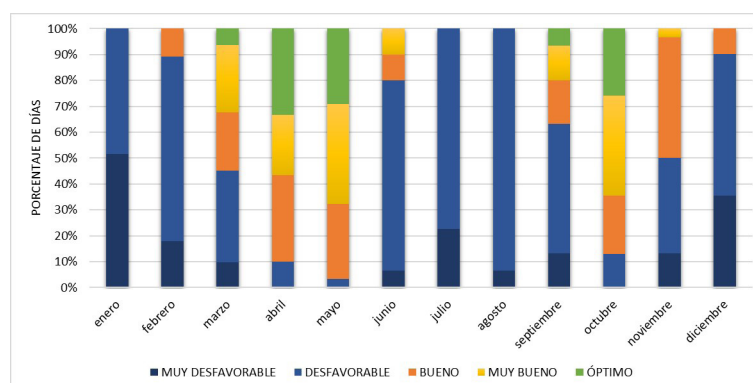
Figura 12. Frecuencia mensual de las categorías de aptitud climático-turística para el escenario 2030 en la ciudad de Granada
