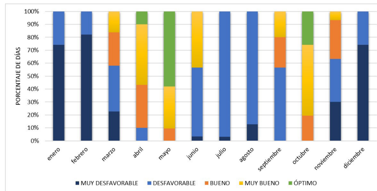
Figura 11. Frecuencia mensual de las categorías de aptitud climático-turística para el escenario actual en la ciudad de Granada
