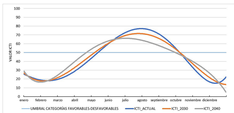
Figura 6. Modelo de simulación de evolución diaria del ICTI para los escenarios 2030/40 en la ciudad de León
