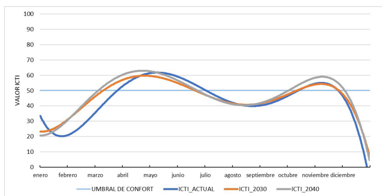
Figura 10. Modelo de simulación de evolución diaria del ICTI para los escenarios 2030/40 en la ciudad de Granada
