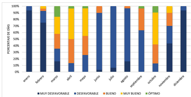
Figura 3. Frecuencia mensual de las categorías de aptitud climático-turística para el escenario actual en la ciudad de Madrid
