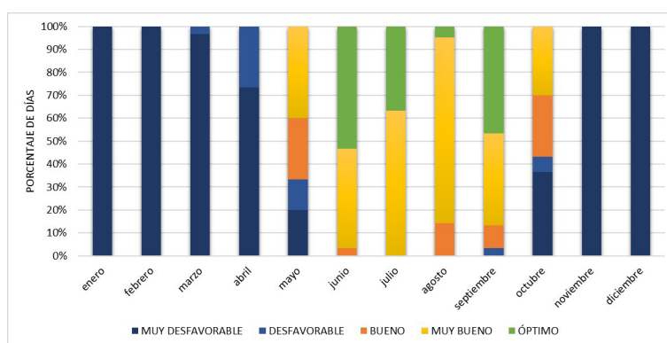
Figura 7. Frecuencia mensual de las categorías de aptitud climático-turística para el escenario actual en la ciudad de León
