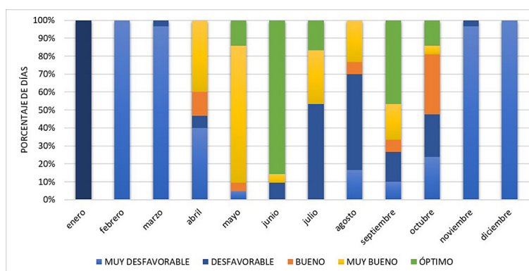
Figura 9. Frecuencia mensual de las categorías de aptitud climático-turística para el escenario 2040 en la ciudad de León
