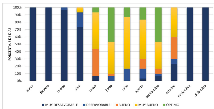
Figura 8. Frecuencia mensual de las categorías de aptitud climático-turística para el escenario 2030 en la ciudad de León
