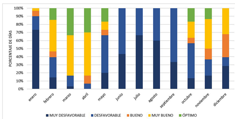
Figura 4. Frecuencia mensual de las categorías de aptitud climático-turística para el escenario 2030 en la ciudad de Madrid
