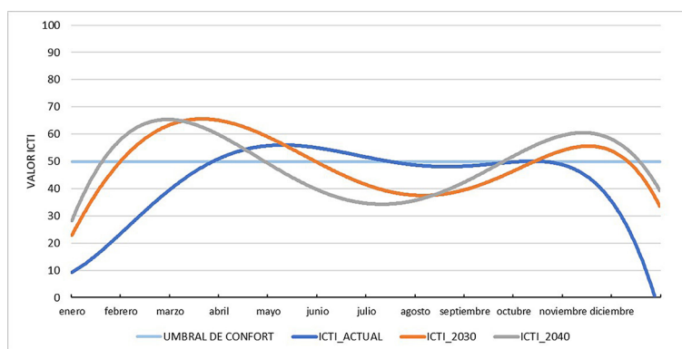
Figura 2. Modelo de simulación de evolución diaria del ICTI para los escenarios 2030/40 en la ciudad de Madrid
