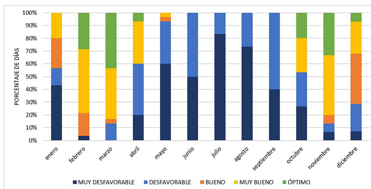
Figura 5. Frecuencia mensual de las categorías de aptitud climático-turística para el escenario 2040 en la ciudad de Madrid
