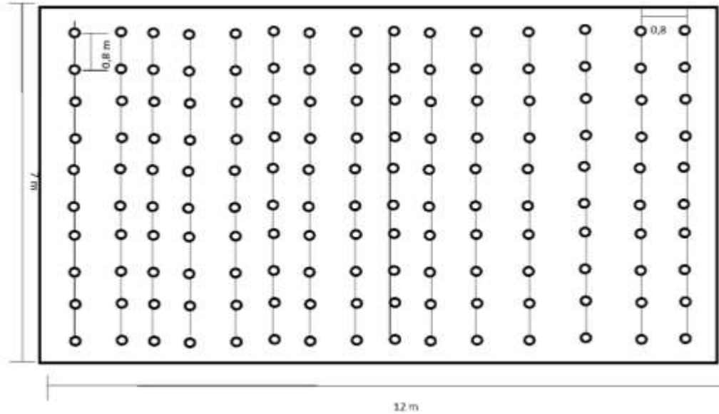
Figura 5: Diseño de la distribución en planta en línea de la huerta urbana en Sierra Morena, Bogotá D.C. Vista Superior.
