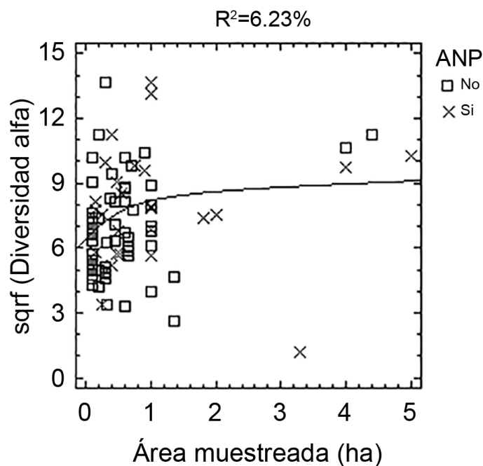
Figura 1: Curva área muestreada-diversidad \alpha ( \sqrt{\text{diversidad } \alpha}=7.00281+0.25244 * \log \text{ área} ) para todas las áreas naturales.
