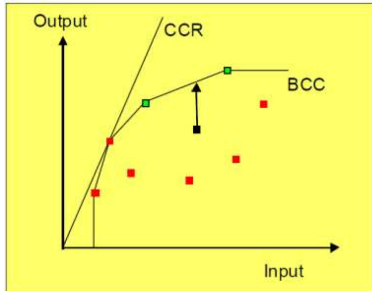
Gráfica 2. Proyección modelos DEA CCR y DEA BCC Outputs Orientados
