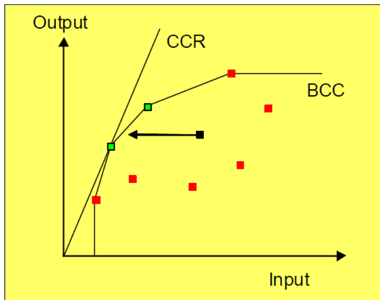
Gráfica 1. Proyección modelos DEA CCR y DEA BCC Inputs Orientados
