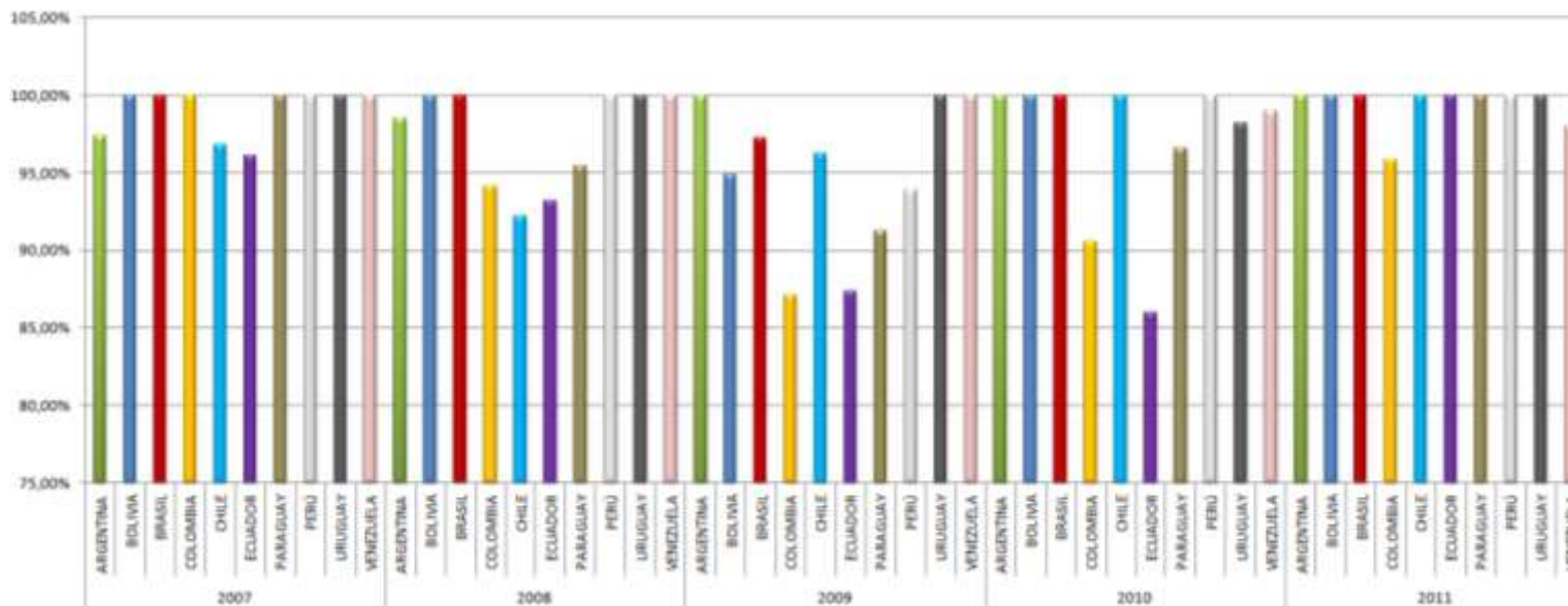
Gráfica 3. Niveles de eficiencia Latinoamérica. 2007 – 2011.
