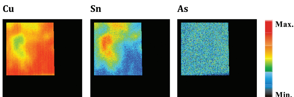
Fig. 14 – Mapas de distribuição elemental do machado 1693/Arq.184 (Herdade do Sobral da Várzea, Santa Cruz) (dimensões aproximadas dos mapas: 0,7 \times 0,8 \text{ mm}^2 ).
