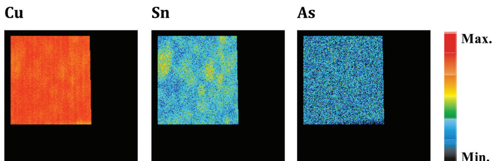
Fig. 12 – Mapas de distribuição elemental do machado 1697/Arq.188 (S. Francisco, Santiago do Cacém) (dimensões aproximadas dos mapas: 0,7 \times 0,8 \text{ mm}^2 ).
