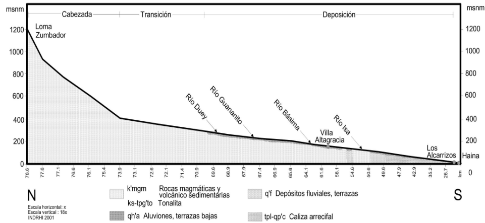
Figura 3 Esquema del perfil longitudinal del Río Haina
