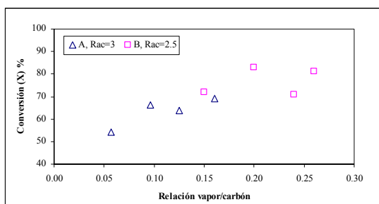
Figura 3. Efecto de la relación vapor/carbón (Rvc) sobre la conversión del carbón
