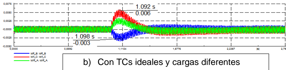
Figura 2. Comportamiento de las componentes RMS en la corriente diferencial con y sin TCs diferentes.
