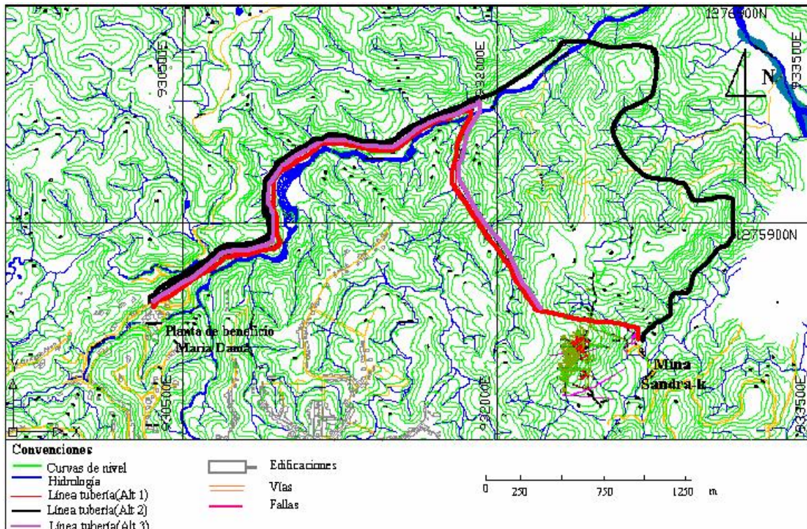
Figura 1. Alternativas de trazados.
