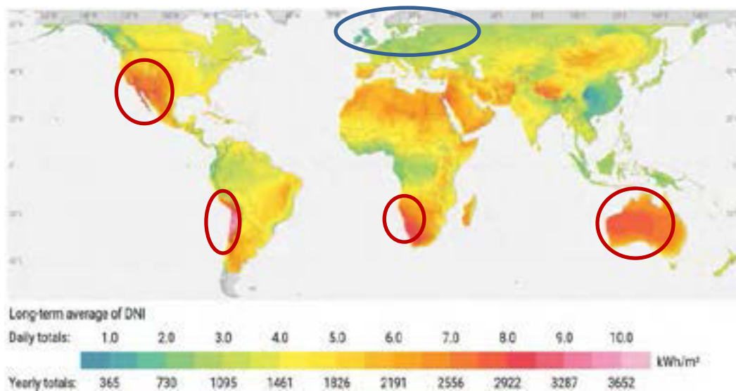
Figura 2. Irradiación normal directa. Fuente:
