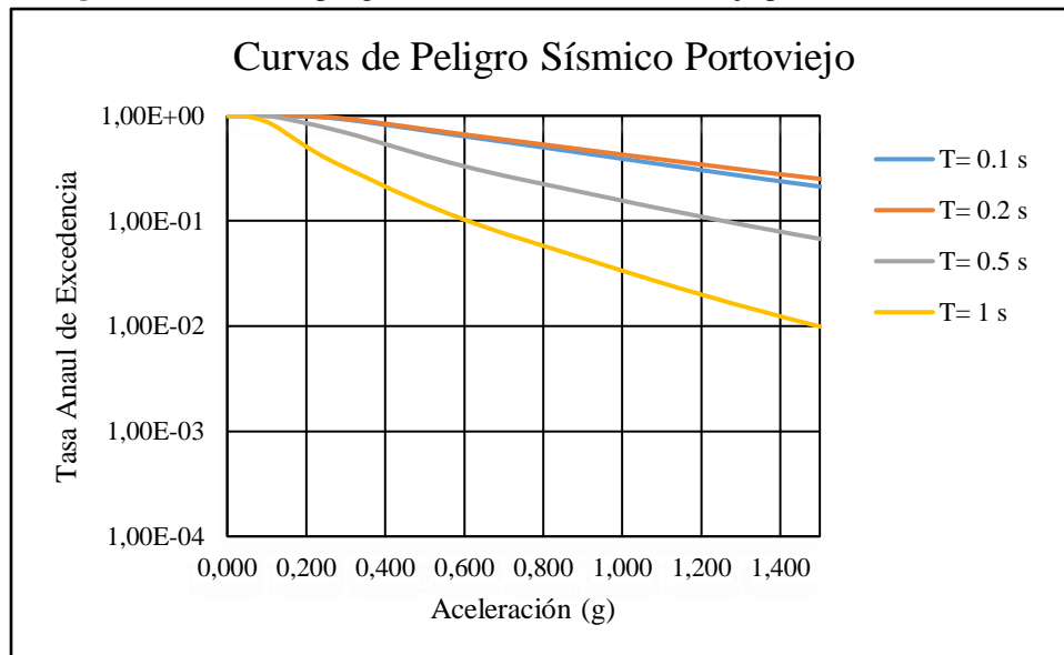
Figura 16: Curvas de peligro sísmico del cantón Portoviejo para fuentes corticales.
