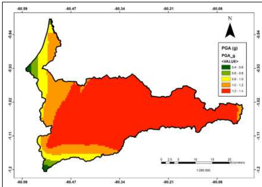
Figura 15.: Mapa de PGA del Cantón Portoviejo para fuentes de subducción en un periodo de retorno de 475 años.
