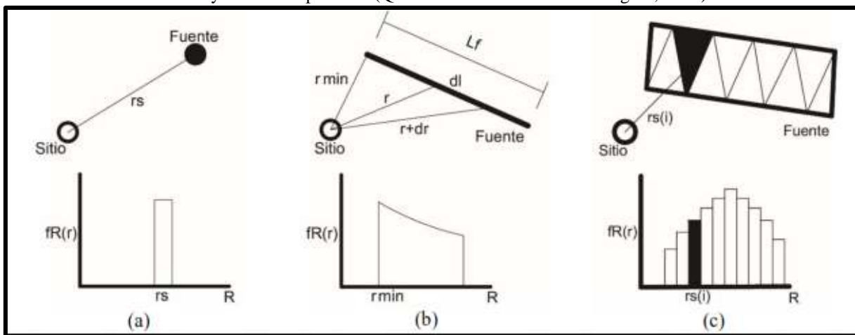
Figura 7: Tipos de fuentes y distancias fuente-sitio. (a) Fuente y distancia puntual, (b) fuente y distancia lineal y (c) fuente y distancia tipo aérea.(Quinde Martínez & Reinoso Angulo, 2016)
