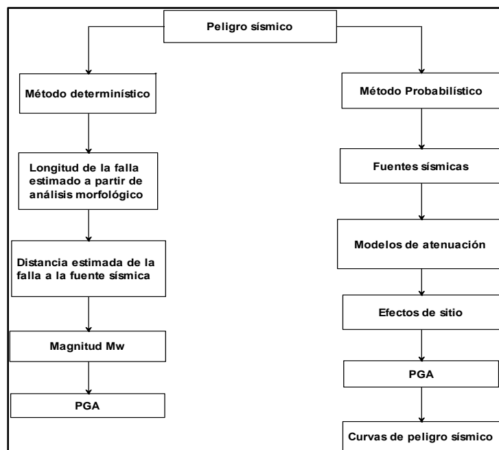
Figura 5: Flujoograma de procesos para el estudio de peligro sísmico.
