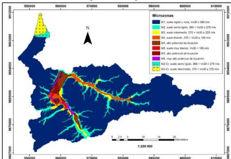
Figura 2: Mapa de microzonificación sísmica del cantón Portoviejo. (Instituto Geofísico IGEPN & Fundación Venezolana de Investigaciones Sismológicas, 2017)
