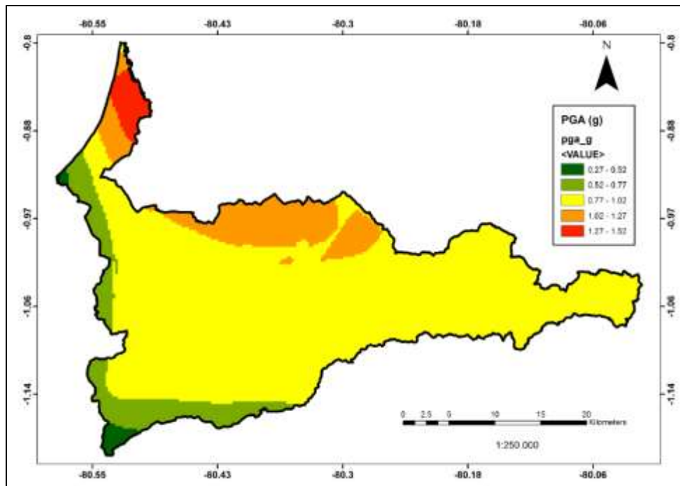
Figura 14: Mapa de PGA del Cantón Portoviejo para fuentes corticales en un periodo de retorno de 475 años.
