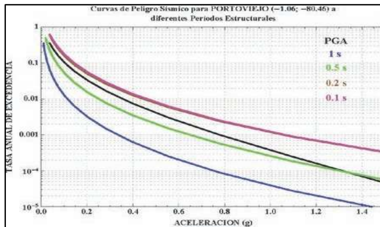
Figura 11: Curvas de peligro sísmico para Portoviejo. (Ministerio de Desarrollo Urbano y Vivienda & Cámara de la Industria y la Construcción, 2015)
