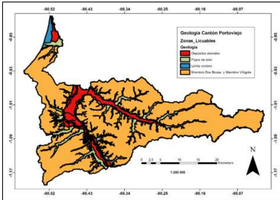
Figura 3: Geología del Cantón Portoviejo. (Instituto Geofísico IGEPN & Fundación Venezolana de Investigaciones Sismológicas, 2017)
