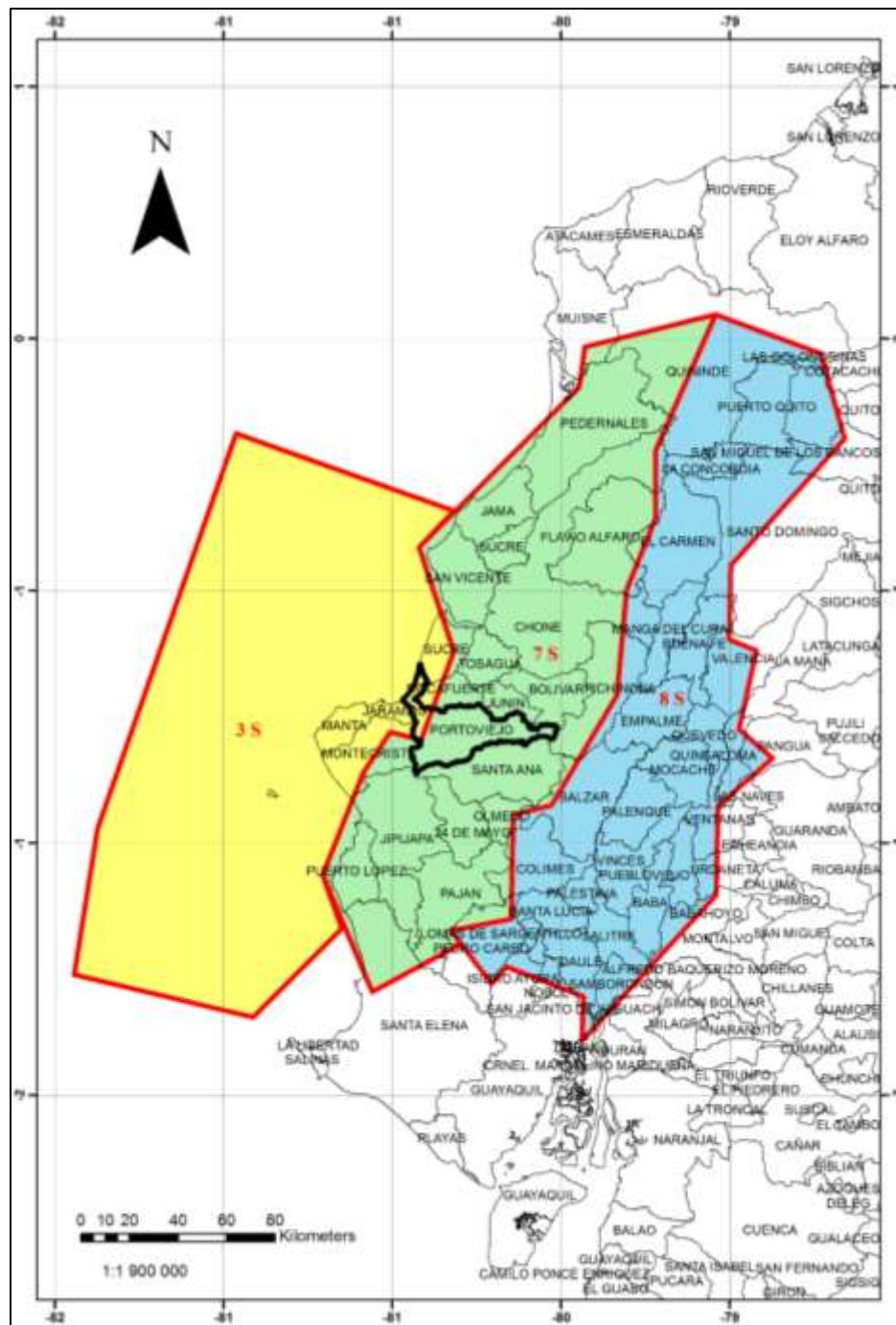
Figura 9: Mapa de bloques de subducción propuestos para el cantón Portoviejo (Chunga, 2010)
