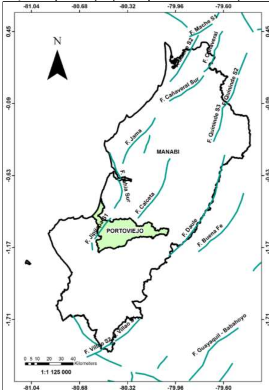
Figura 6: Mapa de fallas geológicas en la provincia de Manabí (Chunga, 2010)
