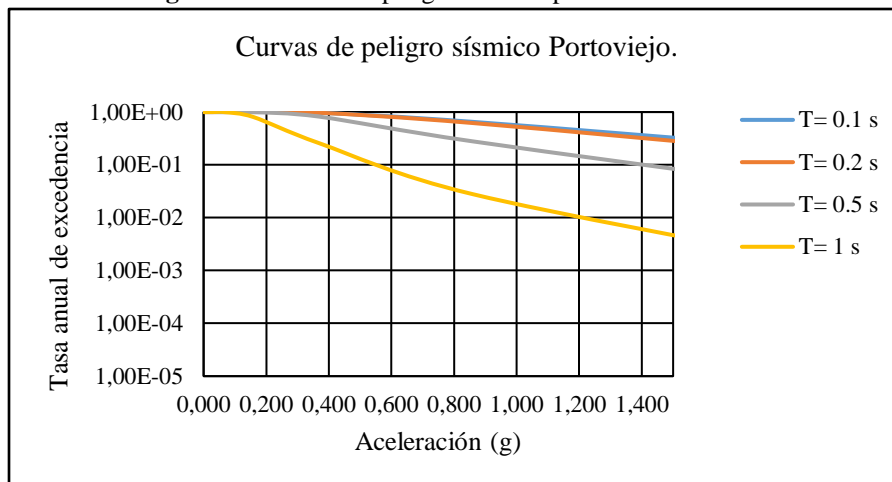
Figura 17: Curvas de peligro sísmico para fuentes de subducción.
