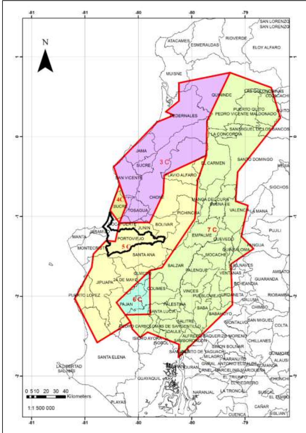
Figura 8: Mapa de bloques corticales propuestos para el cantón Portoviejo (Chunga, 2010)
