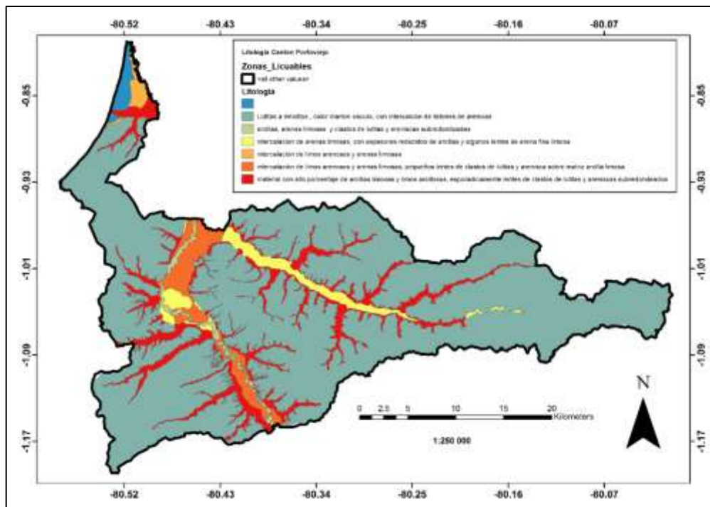
Figura 4: Litología del Cantón Portoviejo. (Instituto Geofísico IGEPN & Fundación Venezolana de Investigaciones Sismológicas, 2017)
