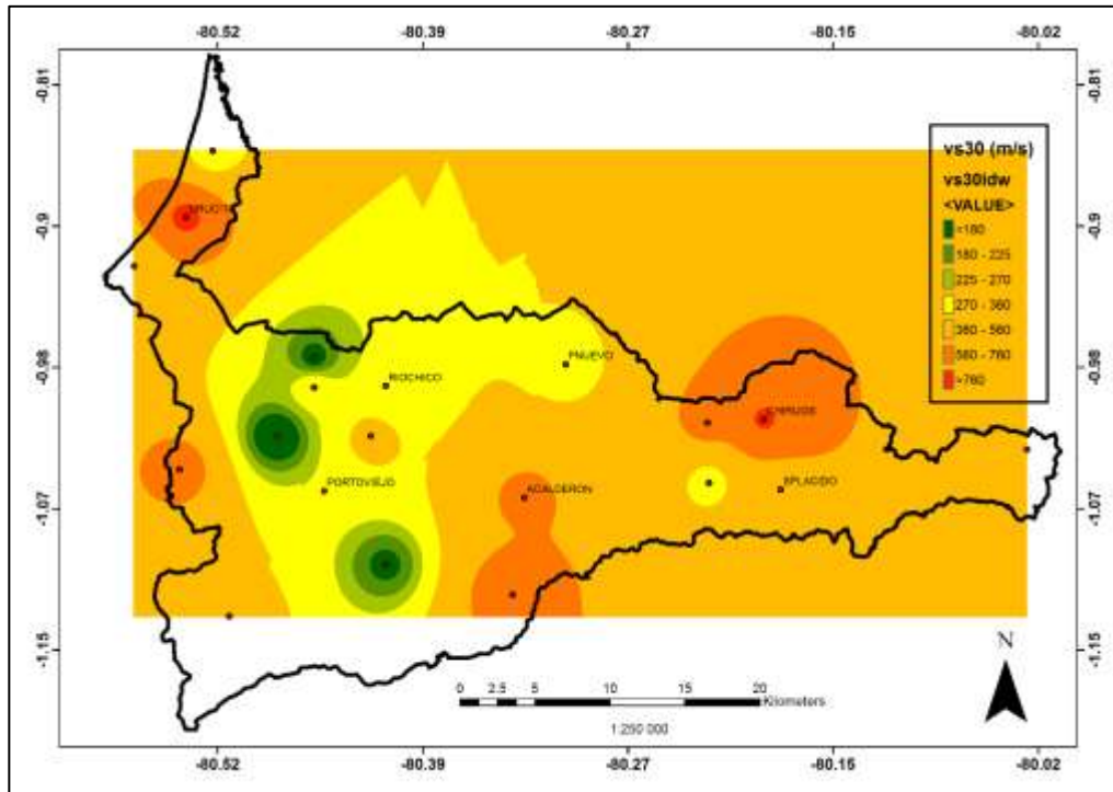
Figura 10: Mapa de vs30 para el cantón Portoviejo a escala 1:250.000 (Instituto Geofísico IGEPN & Fundación Venezolana de Investigaciones Sismológicas, 2017)
