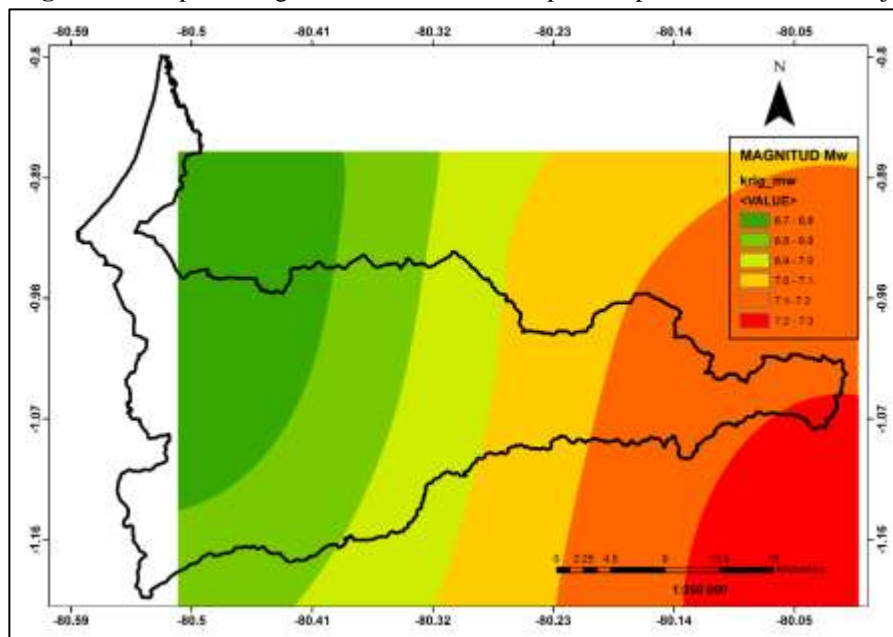
Figura 12: Mapa de magnitudes máximas Mw esperadas para el cantón Portoviejo.
