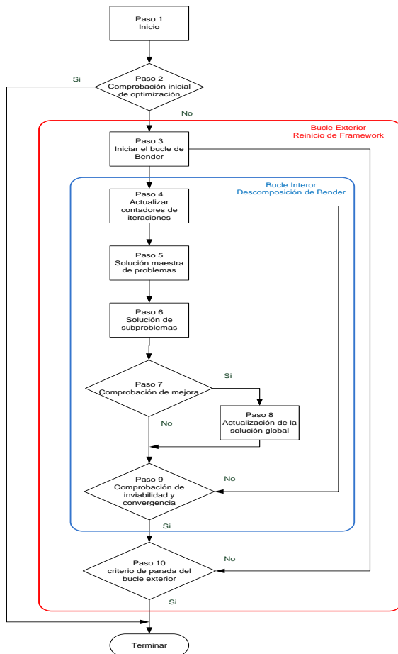
FIG. 1. METODOLOGÍA PROPUESTA CONTRA ATAQUES INTENCIONALES.
