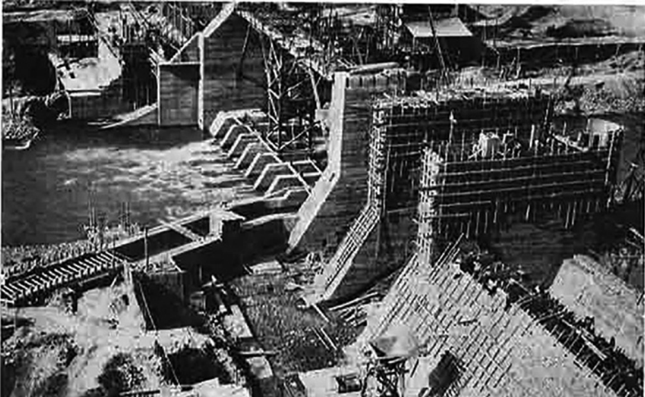
Construcció de la presa de Sant Llorenç. Punt on agafa l'aigua el Canal Auxiliar.
