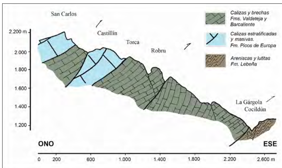
FIG. 9. Corte morfoestructural a través de las cumbres del grupo del Robru, del interfluvio de las canales de San Carlos-Mancorbo. Información reelaborada a partir de IGME: Cartografía Geológica. Geode 50.
