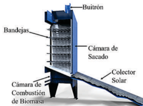
Figura 3. Diseño de secador híbrido solar – Biomasa para frutas. Fuente: elaboración propia.
