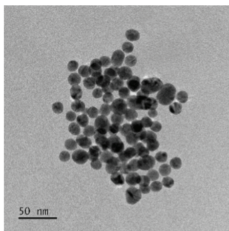
Figura 2 Micrografía de nanopartículas de oro ( 19\pm 5 )* sintetizadas por el método de Turkevich
