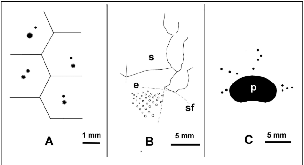
Fig. 2.- Esquemas de la parte proximal del ambulacro III (A); del contacto entre placas esternales y episternales (B), y de la zona peristomial (C); s=esternal, e=episternal; sf=traza dudosa de fasciola subanal; p=peristoma. Del ejemplar n° 85880.1.
