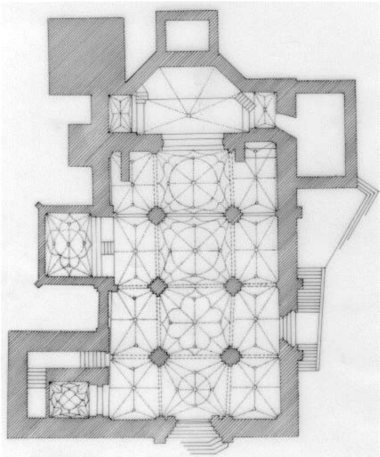
Plano de la Iglesia de Santa María La Mayor, Trujillo
