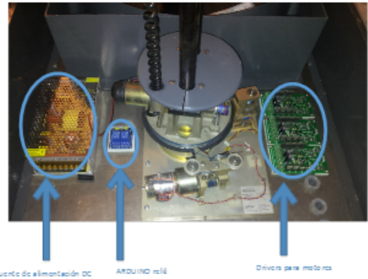
Fig. 8. Instalación de los componentes cercanos al manipulador ZYMARK
