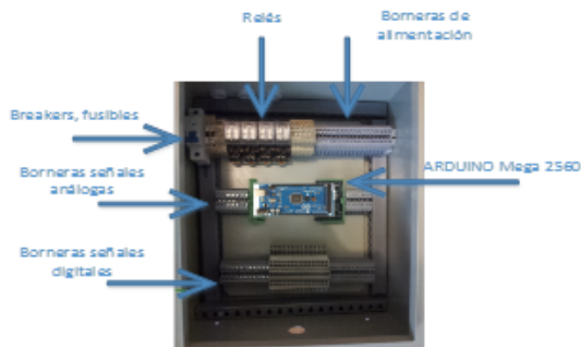
Fig. 11. Disposición de los componentes en el panel de control
