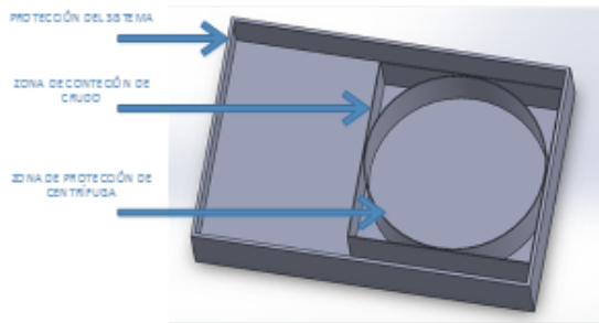
Fig. 5. Diseño de la zona de centrifugación
