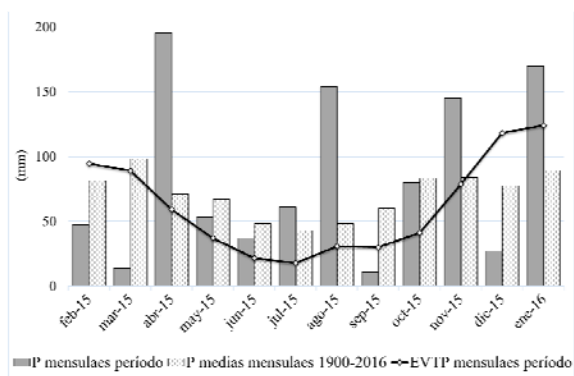
Figura 5. Precipitaciones mensuales históricas y del período de estudio versus evapotranspiración potencial mensual del período.
