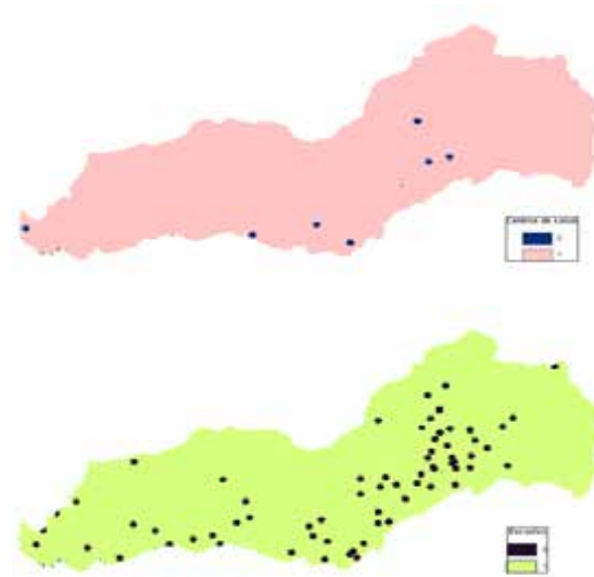
Figura 7. Análisis variable 7 y 8, distancia a centros educativos y centros de salud
