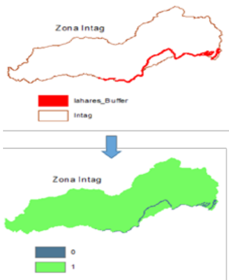
Figura 6. Análisis variable 6, riesgos volcánicos, formación de lahares en la zona de Intag
