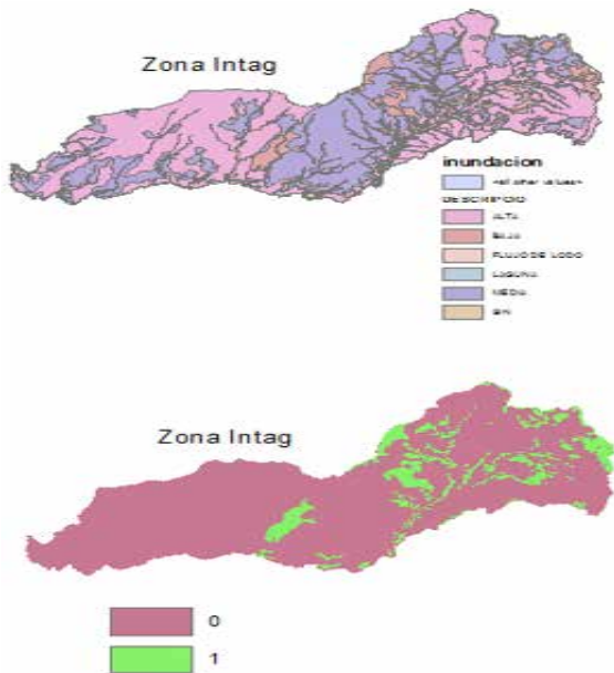
Figura 5. Análisis variable 5, riesgos de inundación y flujos de lodo en la zona de Intag.
