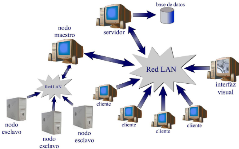
Figura 1. Vista general del sistema de cómputo
