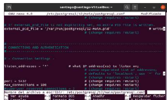
Figura 9. Confirmación de la configuración del postgresql.conf .
