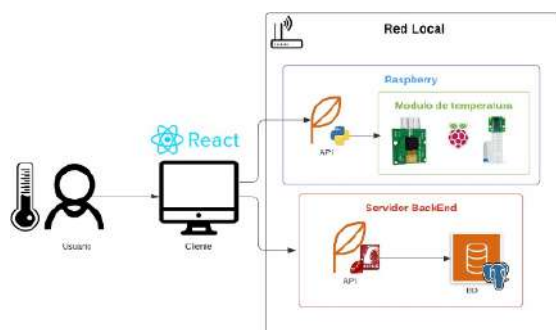
Figura 2. Diagrama Arquitectura del software. Fuente: Elaboración propia
