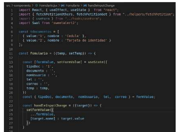
Figura 18. Métodos del componente “ Formulario ” parte 1.
