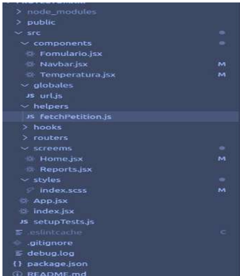
Figura 15. Estructura del proyecto en React.
