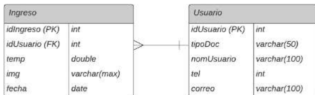
Figura 5. Modelo entidad relación de la base de datos. Fuente: Elaboración propia
