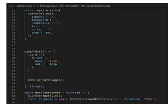
Figura 19. Métodos del componente “ Formulario ” parte 2.
