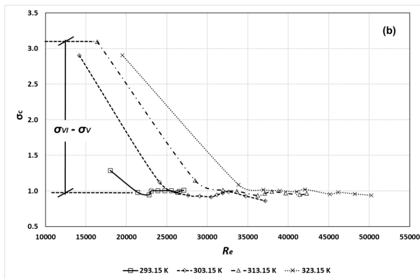
Figura 4. Desarrollo de la cavitación, \sigma_c vs Re .
