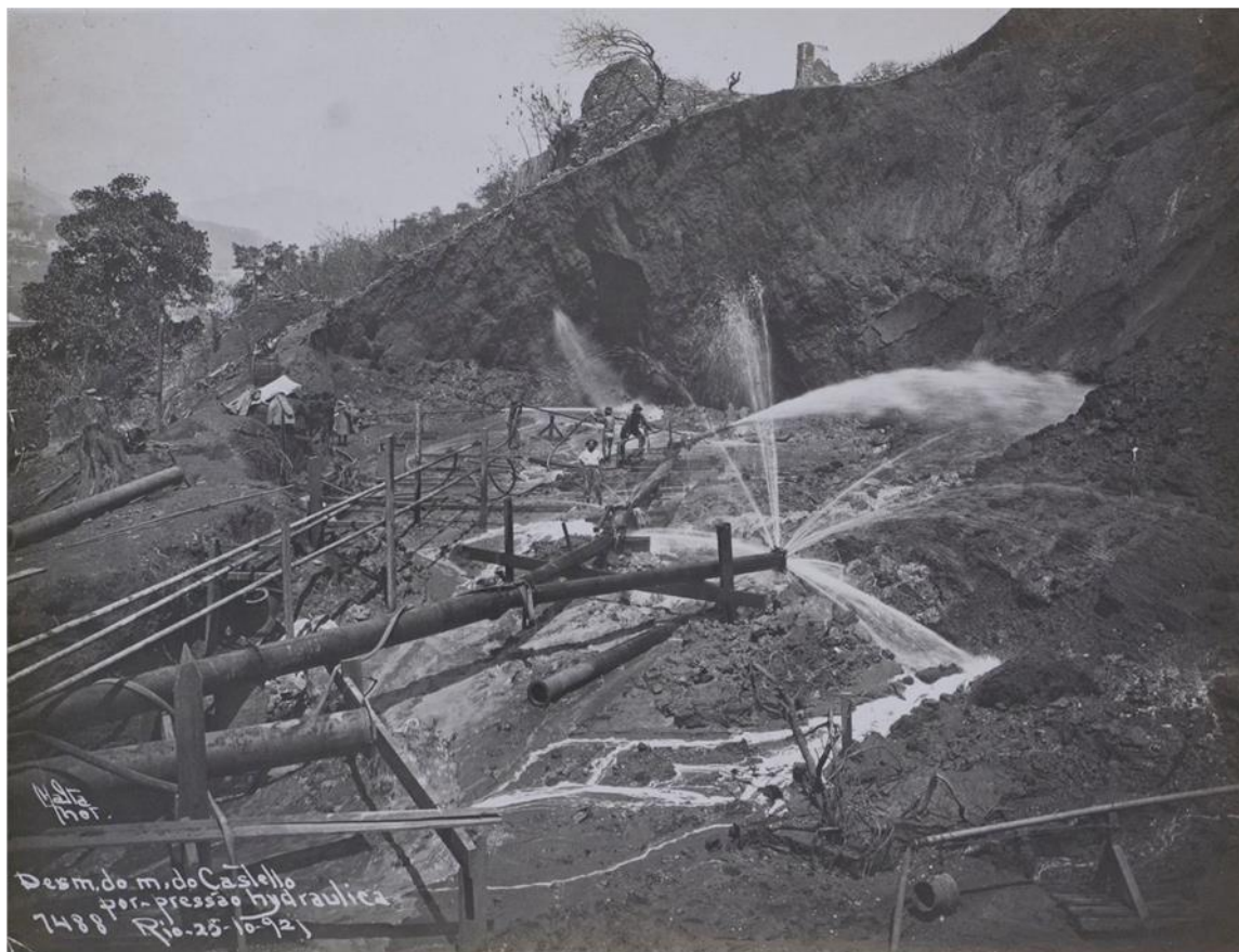
Figura 2 – Obras de desmorte do Morro do Castelo por pressão hidráulica, em 1921.
