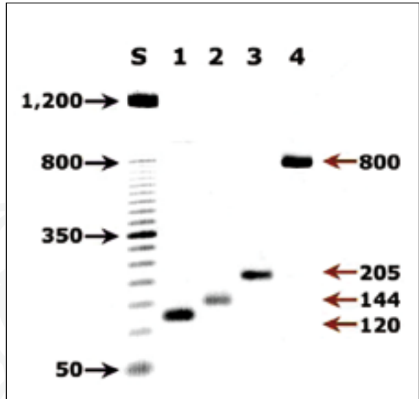
Figura 56. Análisis en gel de agarosa al 2% de una prueba diagnóstica de PCR que identifica el DNA de las diferentes especies de Plasmodium . El carril S muestra el marcador de tamaño molecular. En el carril 1 se observa la banda de 120 pares de bases (bp) que representa P. vivax , en el carril 2 se observa la banda de 144 bp que representa P. malariae , en el carril 3 se observa la banda de 205 pares de bases que representa P. falciparum y en el carril 4 se observa la banda de 800 pares de bases que representa P. ovale .
