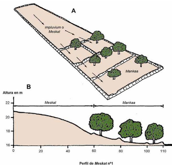
Figura 1. Planta (A) y perfil (B) de los principales elementos del sistema meskat : el meskat en sentido estricto o hamada (sector de captación) y el mankaa (sector de riego)
