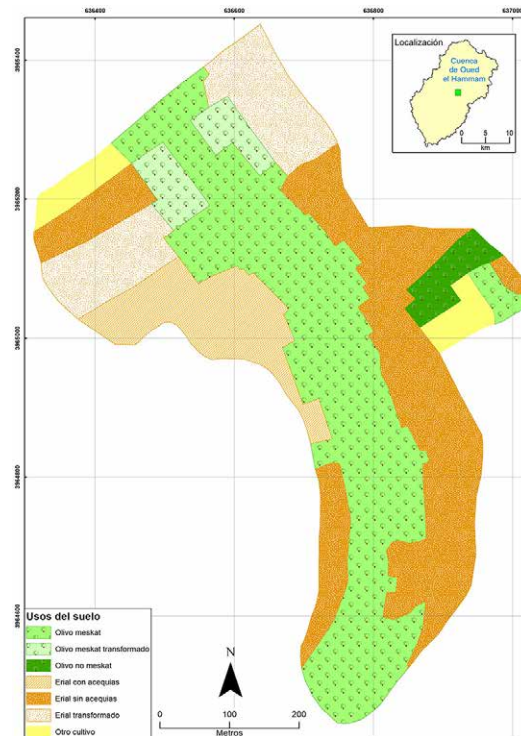
Anexo I. Sistema de meskat en sector de vaguada “As-sabbaghin-Sur”
