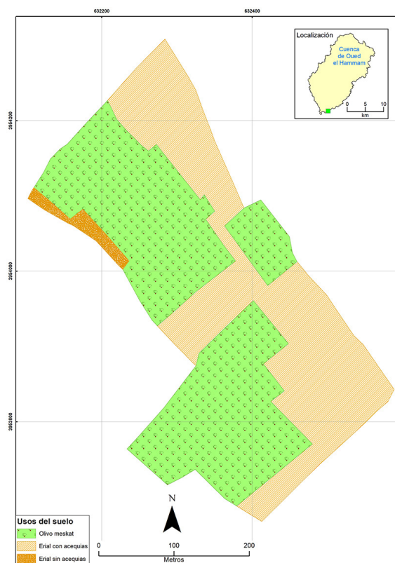
Anexo 9. Sistema de meskat en sector de glaciés “Hanshir Bashir”
