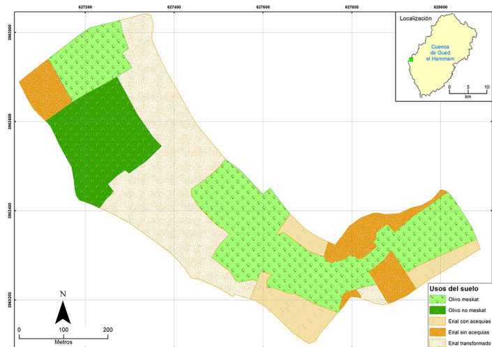
Anexo 14. Sistema de meskat mixto "Hanshir At-tawila-1"
