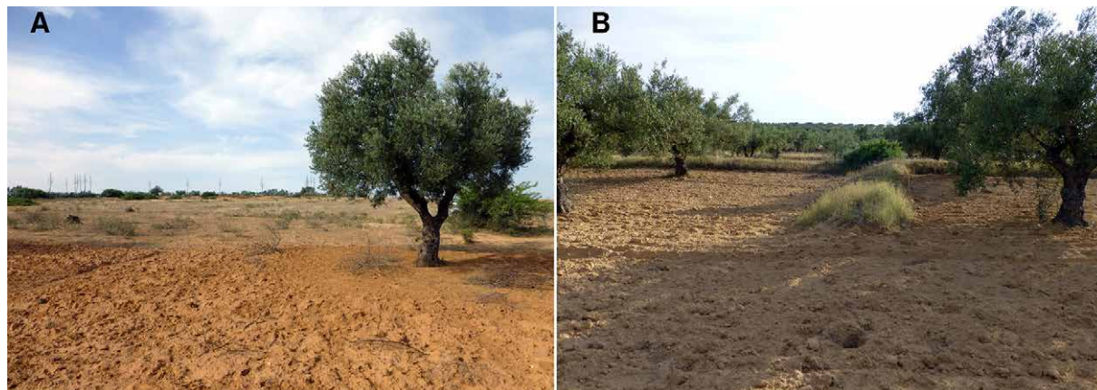
Figura 2. Un sistema de meskat en Oued el Hammam. A) el contacto entre la zona de captación “ meskat ” y la de recepción “ mankaa ”, B) la zona de mankaa donde se observan los primeros compartimentos
