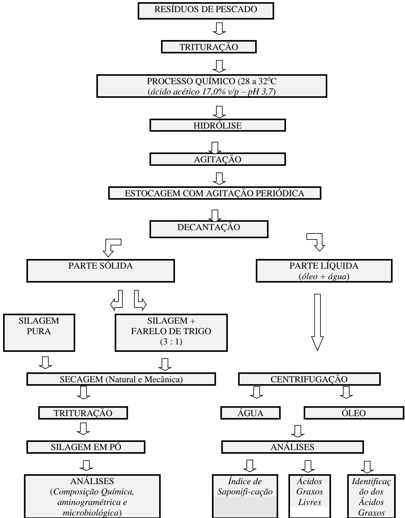
-Fluxograma do processo de obtenção de silagens em pó e óleo de resíduos de pescado.
