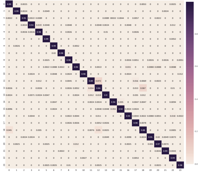
Fig. 5. Confusion Matrix.
