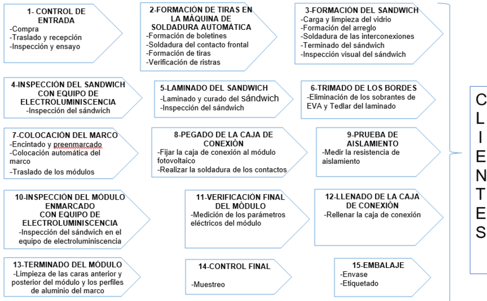
Figura 2. Desagregación de los procesos y subprocesos en la producción de paneles fotovoltaicos.
