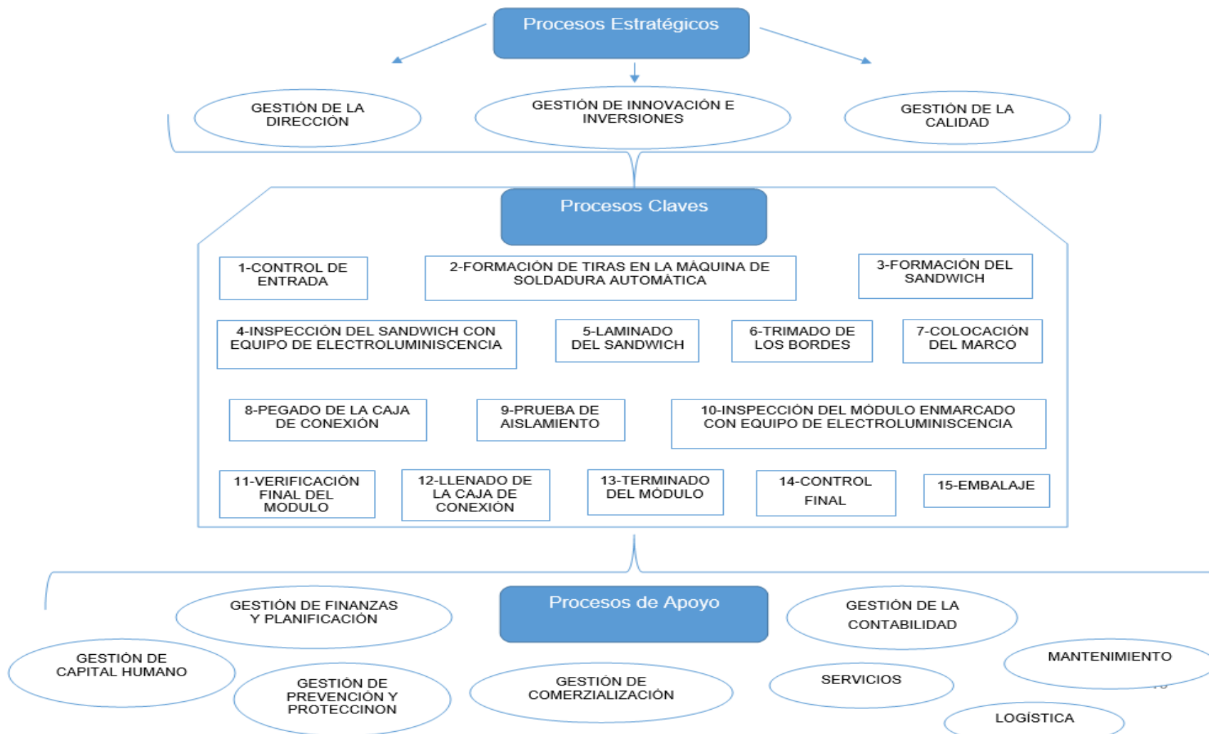
Figura 1. Clasificación de los procesos que intervienen en la creación de valor de la producción de paneles fotovoltaicos.
