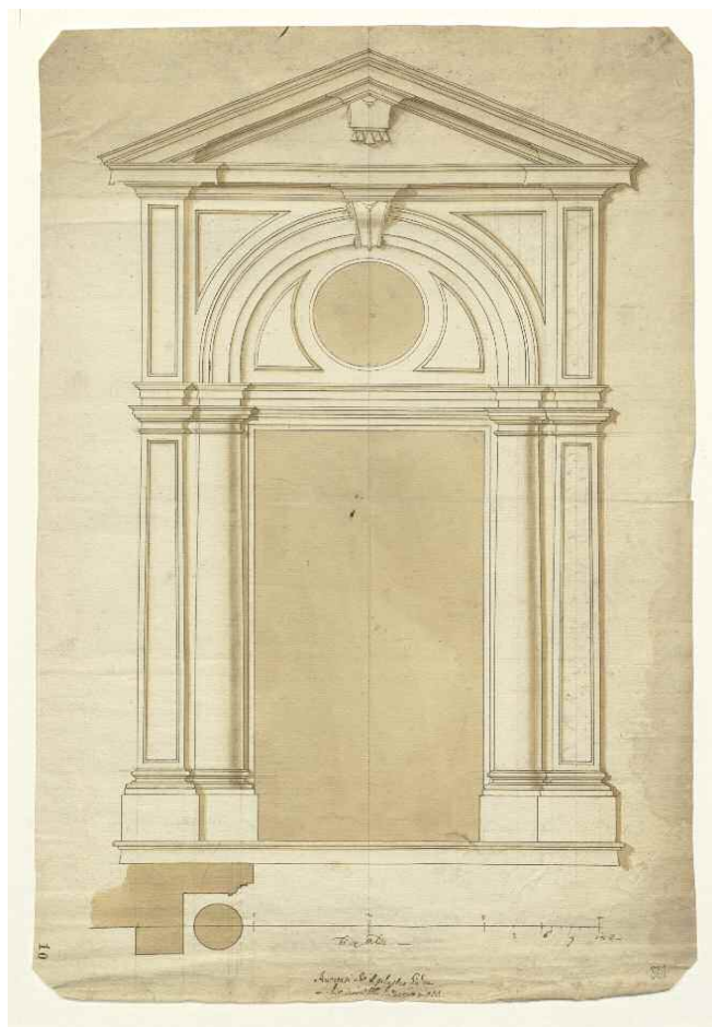
Fig. 4. Bottega di Francesco Maria Ricchino?, portale «cinquecentesco», 272 x 423 mm, matita, penna e inchiostro, inchiostro dilavato/acquarello, (BAMi, F. 251 inf., f. 10). ©Veneranda Biblioteca Ambrosiana / Mondadori Portfolio.
