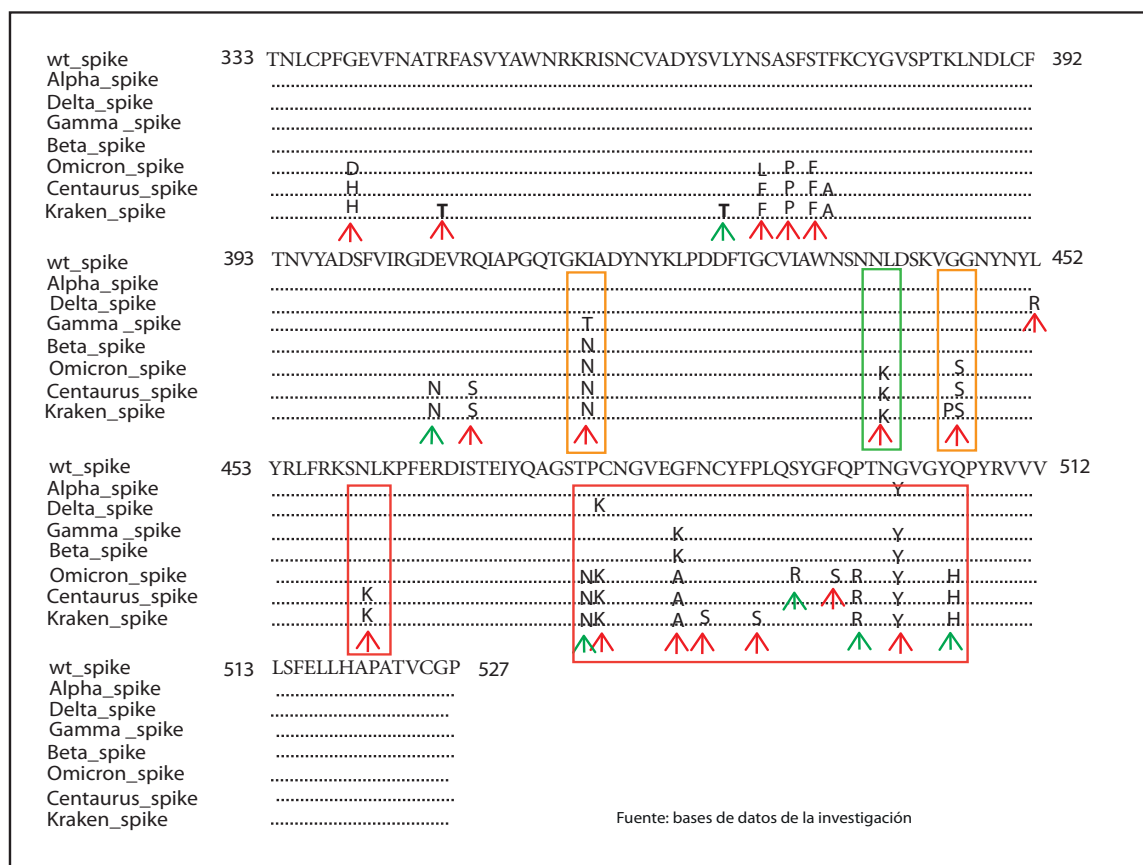
Figura 1. MSA de la secuencia del RBD (333-527aa) de SARS-CoV-2 wt y las diferentes variantes de importancia clínica. Las mutaciones sinónimas y no sinónimas están señaladas con flechas verdes y rojas, respectivamente. Recuadro rojo: secuencia de interacción con IgG-antiRBD. Recuadro anaranjado: Sustituciones que producen impedimentos estéricos. Recuadro verde: sustituciones que mejoran la unión con ACE2 (Elaboración propia a partir de la base de datos del NCBI y el software Mega6).
