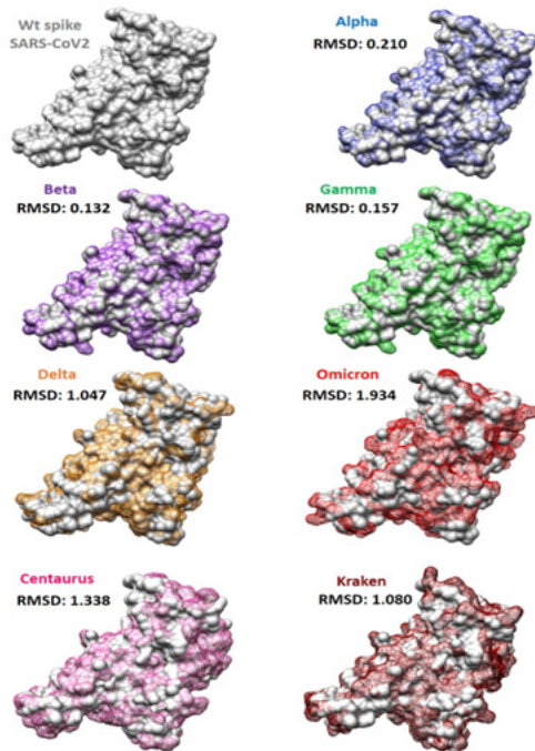
Figura 2. Alineamiento Estructural entre RBD de SARS-CoV2wt (la primera cristalizada en Wuhan) y las diferentes variantes (Elaboración propia a partir de la base de datos PDB y el software Chimera1.15).
