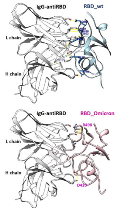
Figura 3. Puentes de H2 (líneas amarillas) en la interacción de IgG-antiRBD con RBD de SARS-CoV-2wt y omicron (Modelo de cintas) (Elaboración propia, PDB: 6xc2, software Chimera).
