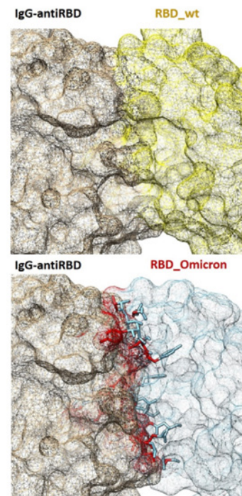
Figura 4. Impedimentos estéricos y posibles choques atómicos (rojo) en la interacción de IgG-antiRBD con RBD de SARS-CoV-2wt y omicron (Modelo de superficie molecular) (Elaboración propia, PDB: 6xc2, software Chimera).
