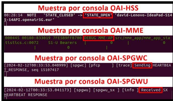
Fig. 3. Funcionamiento del CN. Fuente: Elaboración propia.
