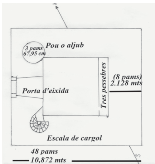
Il·lustració 6. Plànol primera planta de la Torre del Pinaret.
