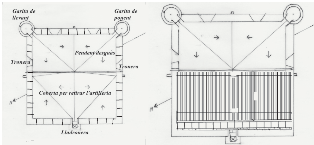
Il·lustració 8. Plànols de la coberta de la Torre del Pinaret.
