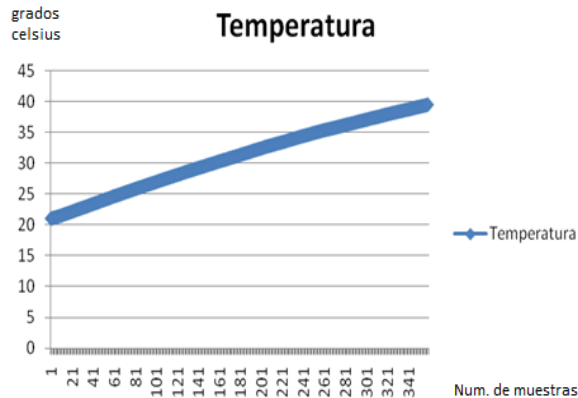
Figura 22.9 Gráfica mostrando la temperatura de los colorantes en el sitio de las pruebas
