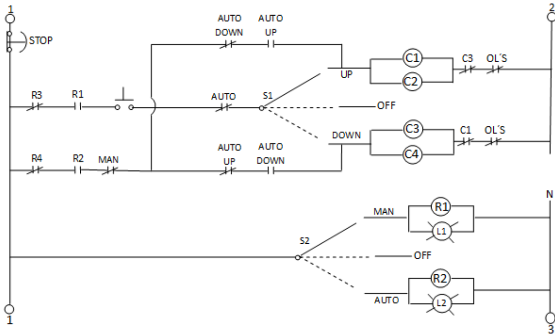
Figura 28.10 Diagrama eléctrico de fuerza y control de la etapa de potencia
