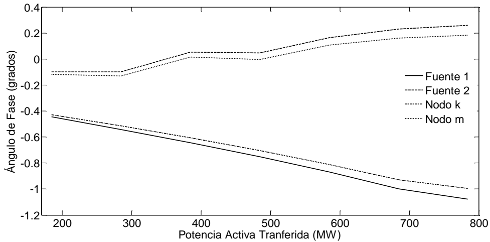
Figura 15.3 Ángulos de fase de las fuentes y nodos en función de la transferencia de potencia activa
