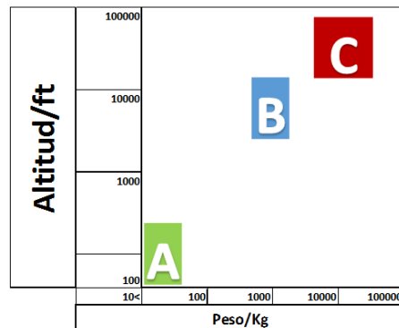
Figura 9.1 Clasificación de los UAVs según la normativa de la EASA [5]
