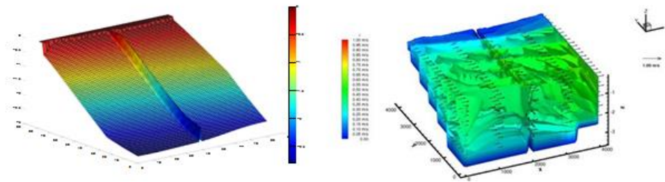
Figura 4.4 Malla 3D de la zona de estudio con campo hidrodinámico con oleoducto
