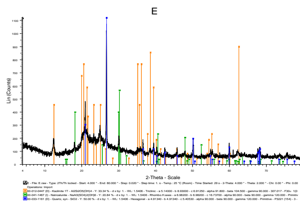
Figura 25 Difractograma de la muestra E, donde se pueden apreciar la amorfización de este caolín
