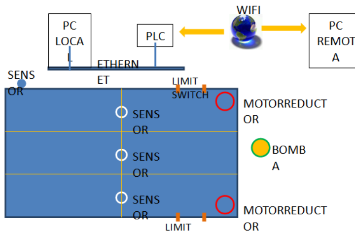
Figura 28.3 Diagrama esquemático de elementos de control climático
