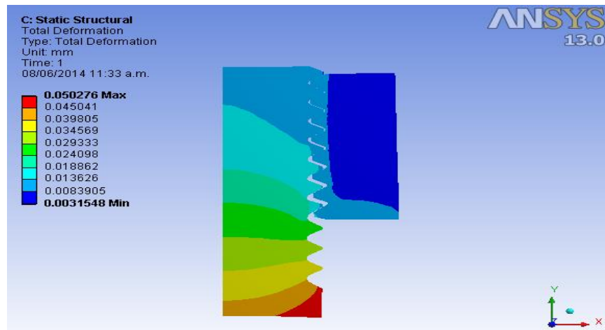
Figura 26.11 Deformación sufrida por la carga aplicada en el contacto tornillo-tuerca.
