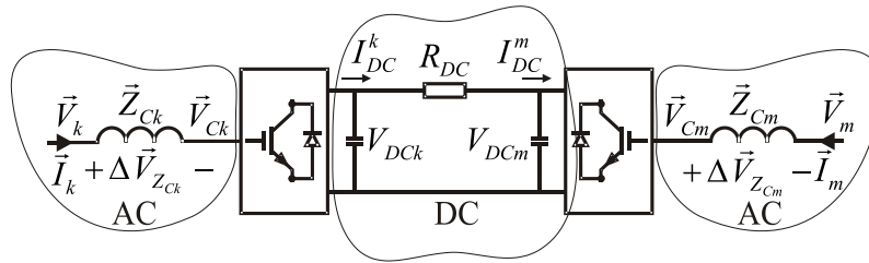
Figura 15 Enlace de transmisión VSC-HVDC
