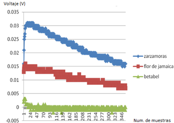
Figura 22.8 Gráfica mostrando los voltajes de los colorantes utilizados
