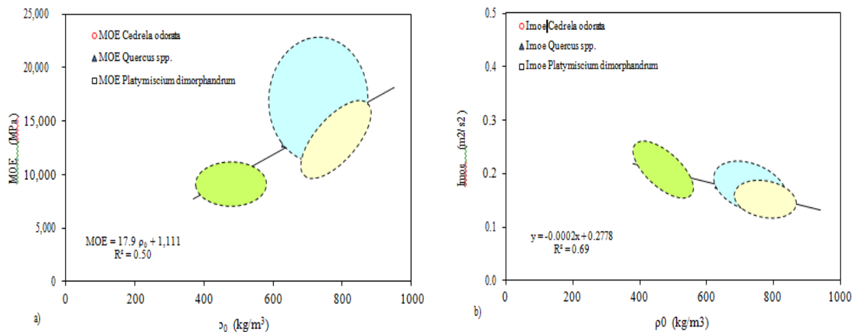
Figura 10.6 Distribuciones y agrupamientos. a) del módulo de elasticidad (MOE) y b) del índice material de elasticidad en flexión ( Imoe ), ambos parámetros en función de la densidad básica \rho_0 de la madera de Cedrela odorata , Quercus spp. y Platymiscium dimorphandrum . Las líneas representan las regresiones entre MOE y \rho_0 e Imoe y \rho_0 , considerando las 96 probetas observadas. R^2 es el coeficiente de determinación con un 95 % de confianza.
