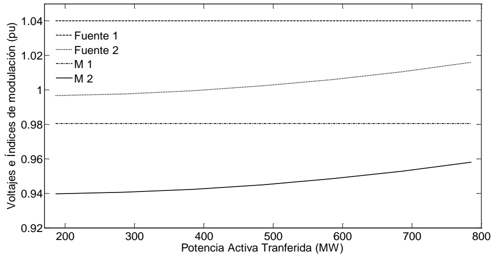
Figura 15.4 Voltajes e índices de modulación en función de la potencia activa transferida con una R_{CD} de 0.001 pu
