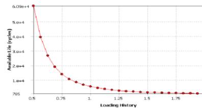
Figura 16.3 Gráfico de resultados del factor de seguridad a la fatiga
