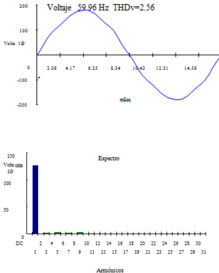
Figura 11.4 Forma de onda de voltaje medida en un tomacorriente
