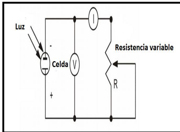
Figura 22.3 Diagrama del circuito para la evaluación de la celda DSSC (Sekar y col., 2010)
