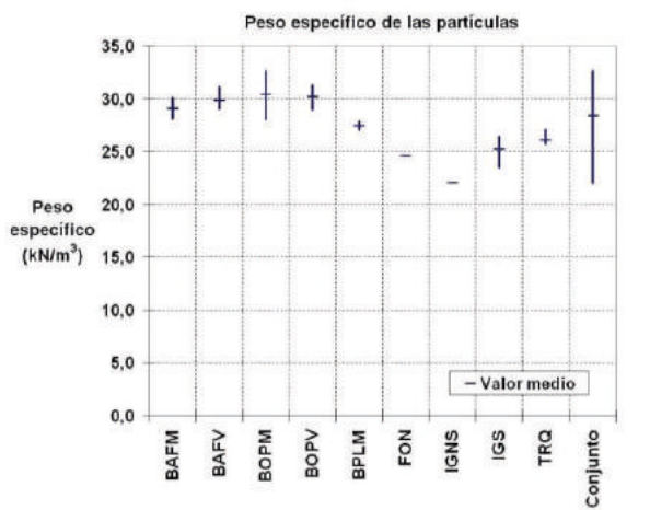
Figura 4. Peso específico real por litotipos: valor medio y rango de variación.
