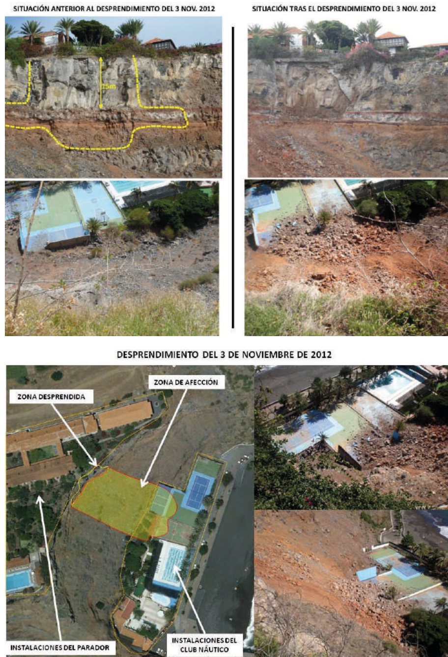
Figura 7. Esquema del desprendimiento del 3 de noviembre de 2012.
