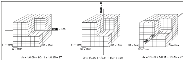
Figura 2. Ejemplo de tres sondeos con RQD de 0 a 100 y J_v=27 (Arlid Palmstrom, 2005).
