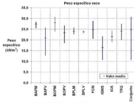
Figura 2. Peso específico seco por litotipos: valor medio y rango de variación.
