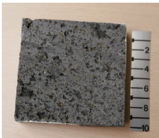
Figura 5. Muestra de mano de basalto olivínico piroxénico masivo (BOPM).
