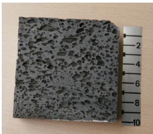
Figura 3. Muestra de mano de basalto afanítico vacuolar (BAFV).
