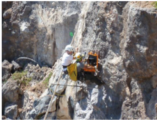
Figura 15. Auscultación de las perforaciones mediante videocámara.
