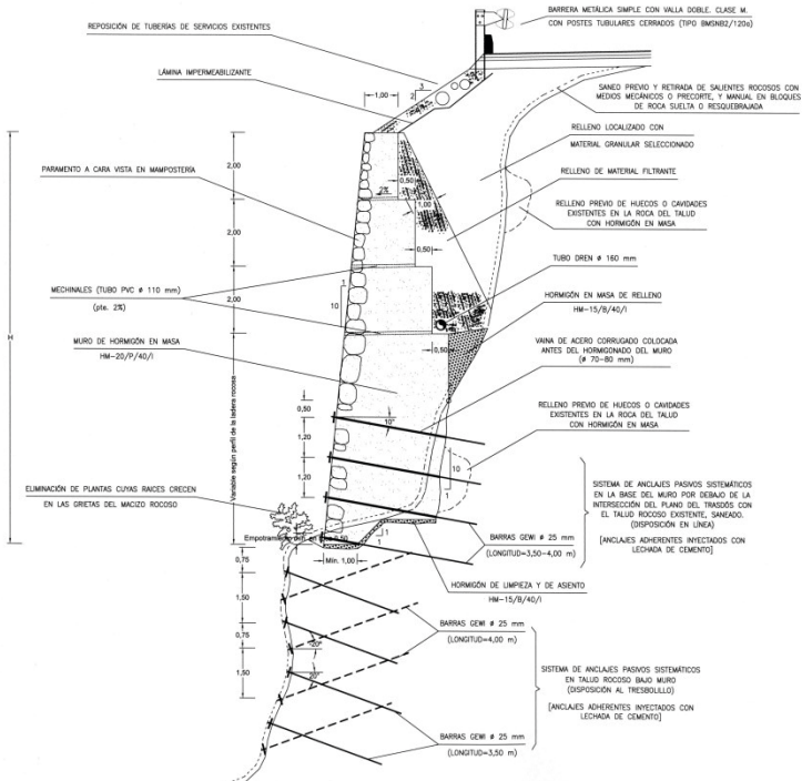
Figura 5. Sección transversal tipo del muro de sostenimiento con anclajes en su base y sistema de cosido del talud rocoso inferior.
