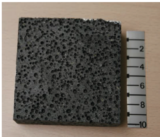
Figura 7. Muestra de mano de basalto olivínico piroxénico vacuolar (BOPV).
