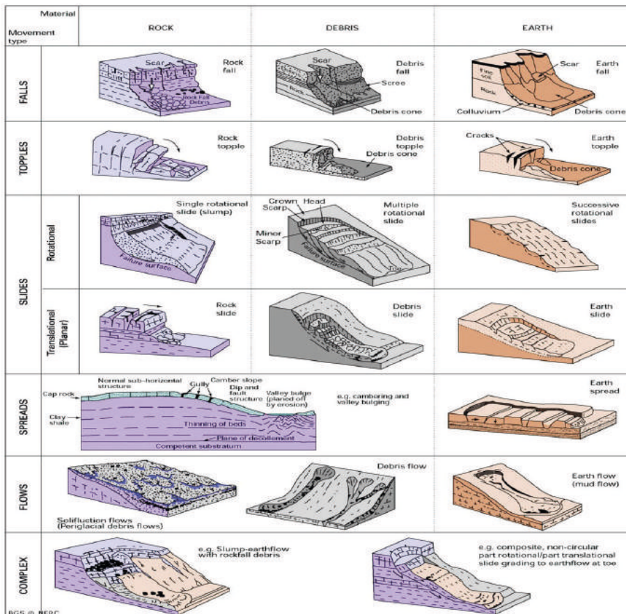
Figura 1. Clasificación de Varnes (1978) de movimientos del terreno.
