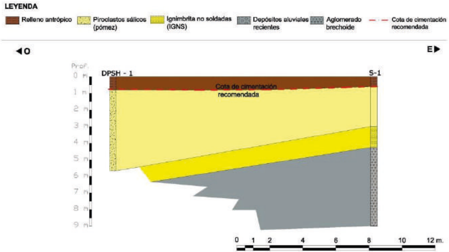
Figura 4. Corte geológico geotécnico en el que se aprecia el elevado espesor que presentan los depósitos piroclásticos sálicos o pómez.
