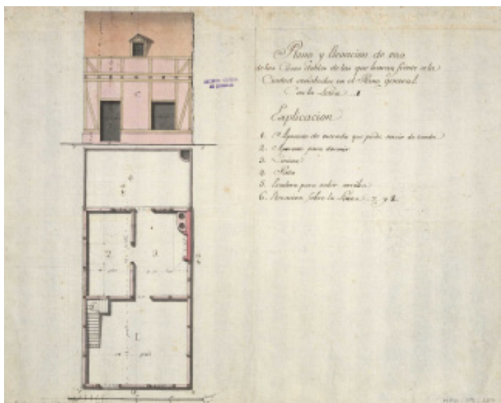
FIG 6. Proyecto de casa de segunda clase del barrio de la Playa, siguiendo las instrucciones de Jorge Próspero Verboom de 8 de septiembre de 1718.
