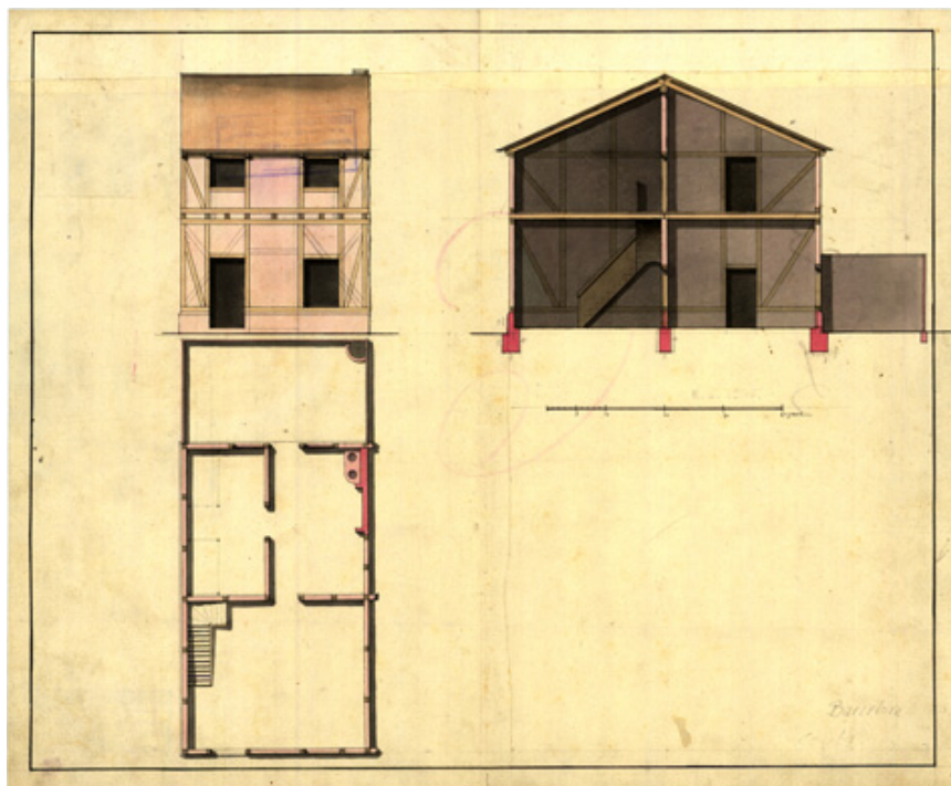
FIG. 4. Proyecto de casa de segunda clase del barrio de la Playa, siguiendo las instrucciones de Jorge Próspero Verboom de 8 de septiembre de 1718.
