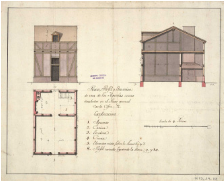
FIG 5. Proyecto de casa de primera clase del barrio de la Playa, siguiendo las instrucciones de Jorge Próspero Verboom de 8 de septiembre de 1718.
