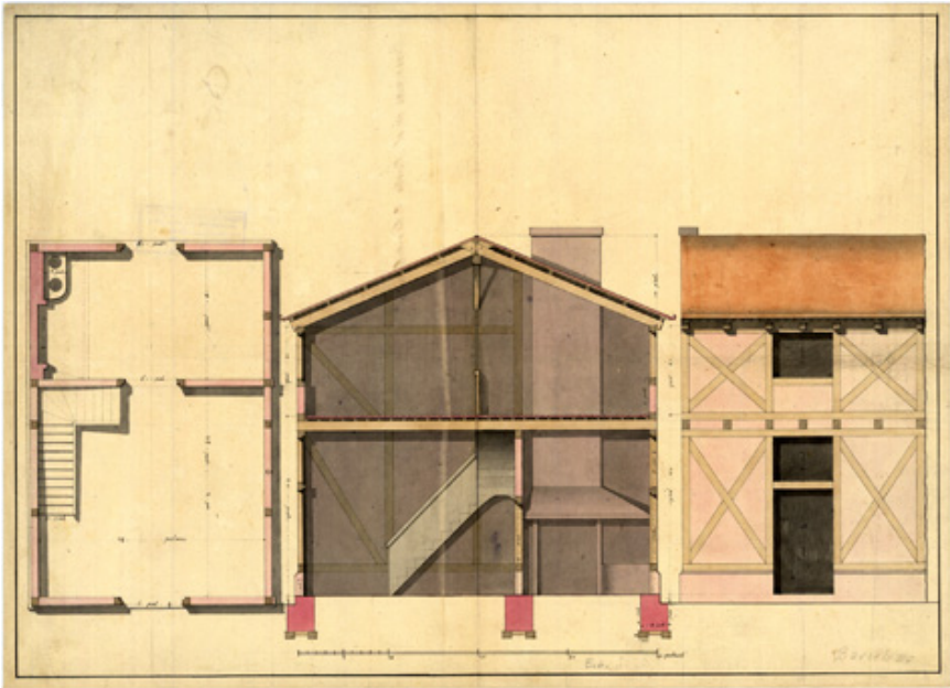
FIG. 3. Proyecto de casa de primera clase del barrio de la Playa, siguiendo las instrucciones de Jorge Próspero Verboom de 8 de septiembre de 1718.
