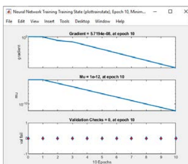
Figura 12. Gráfico del Estado de entrenamiento
