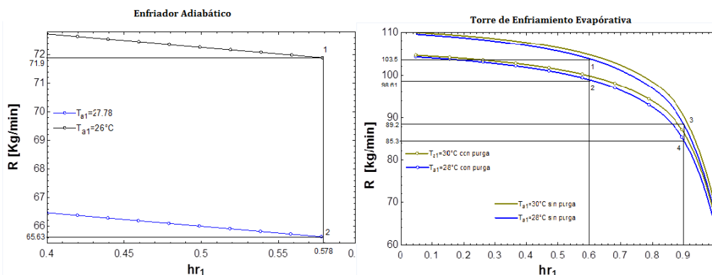
Figura 6. Comparativo del Flujo másico de agua [R] entre la torre de enfriamiento evaporativa, el enfriador adiabático y el Aero-enfriador. R \left[ \frac{\text{Kg}}{\text{min}} \right] vs Humedad [\text{hr}_1]
