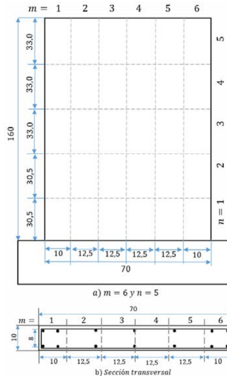
Figura 4. Discretización Especimen W1
