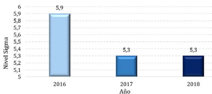
Figura 2334. Nivel Sigma General del Proceso
