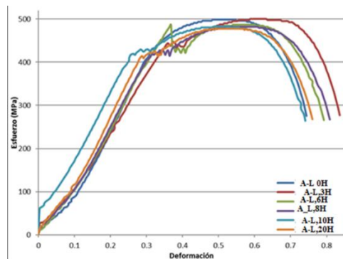
Figura 6. Curvas esfuerzo deformación de acero tipo A cortes longitudinales
